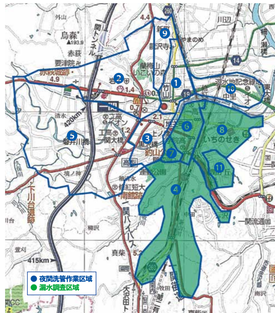
図1 夜間洗管作業区域と漏水調査区域
